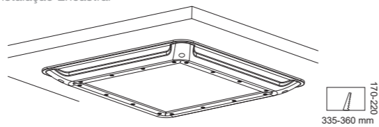
Instalación Empotrado Instalação Encastrar
